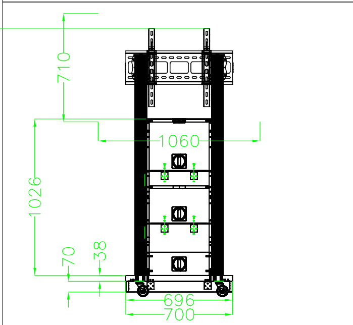
VCM-517-3 Standfuss mit Sockel 700x1754x700
